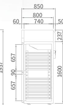
SIDE VIEW (BUN PAN)
